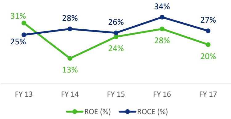
ROE (%) & ROCE (%)
